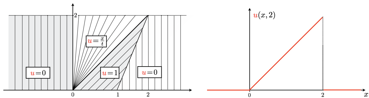
FIGURE 2.21 – Pour u_1 = 0 , u_2 = 1 et u_3 = 0 . La solution pour t \leq t^* = 2 (gauche). Graphe à t = 2 (droite)
