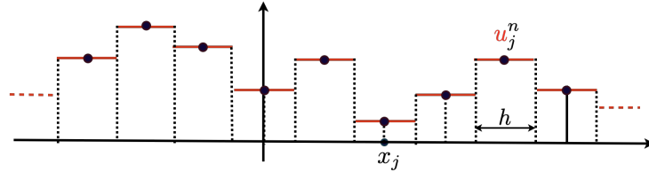
FIGURE 4.7 – La fonction constante par morceaux u^n définie à partir de \{u_j^n, j \in \mathbb{Z}\}
