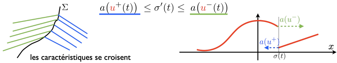
FIGURE 2.12 – Si f est convexe ou concave, en tout temps, le long des chocs entropiques, la vitesse de l'information en amont a(u^-(t)) est supérieure à la vitesse du choc \sigma'(t) elle-même supérieure à la vitesse aval a(u^+(t)) .
